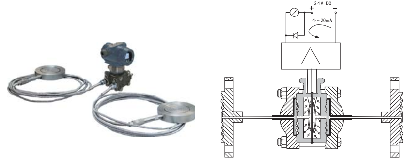
结构原理图
