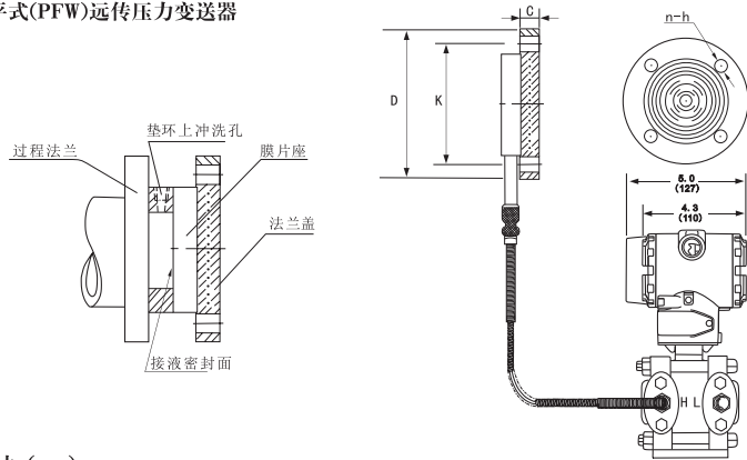
法兰尺寸 (mm)
