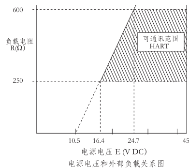
电源电压和外部负载关系图
