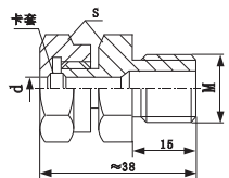
固定卡套
