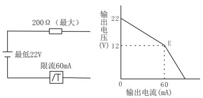
60mA输出时内部等效电路
