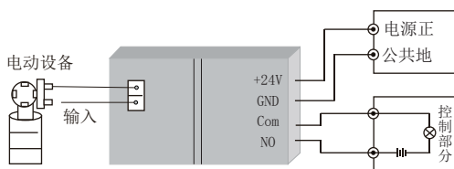
接线图一
