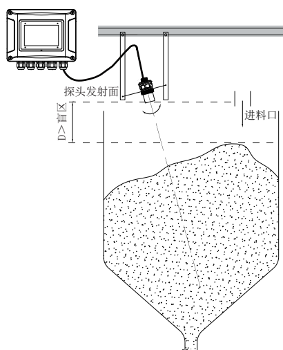
图十三 安装在龙门框
