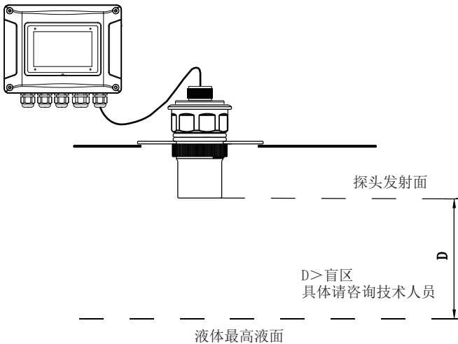
图四 法兰型安装在无接管平顶罐上
