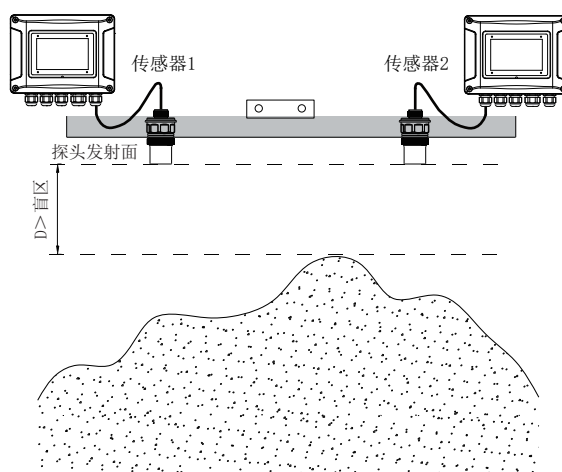
图十四 安装在露天料堆一起重架上
