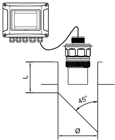
图十六 不浸泡在介质里的延长接管
