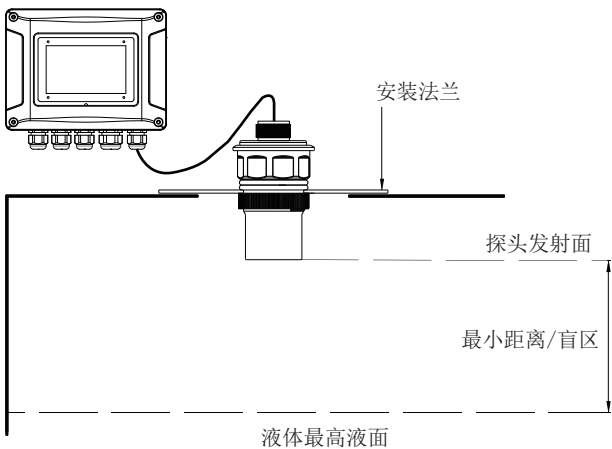
图三 法兰型（锁紧法兰）—安装在平顶罐上
