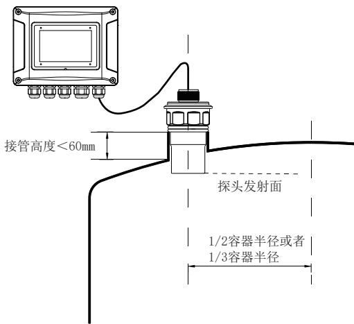
图六 安装在螺纹接管上--拱形罐顶
