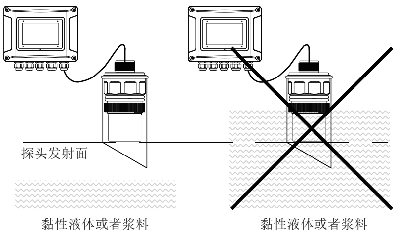
图十五 接管不能浸泡在粘附性介质里
