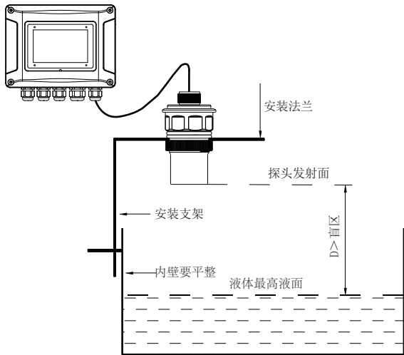
图八 安装在开口容器上一顶部靠一侧支架
