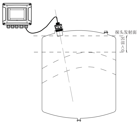
图十二 安装在螺纹接管
