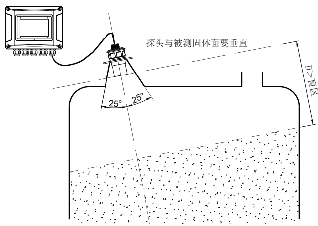
图十七 测量固体介质的延长接管
