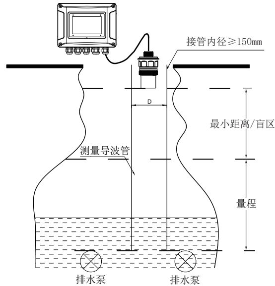
图十 安装在排水井—接管和测量套管
