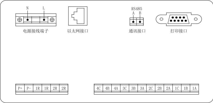
配线说明
