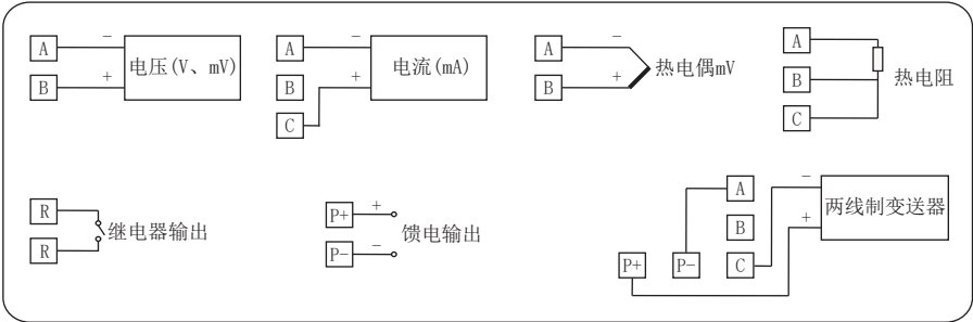
配线说明
