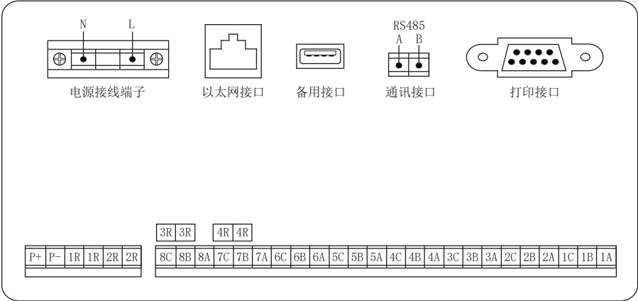
配线说明
