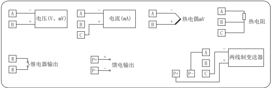
配线说明
