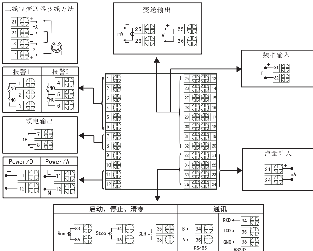
NHR-6661接线图
