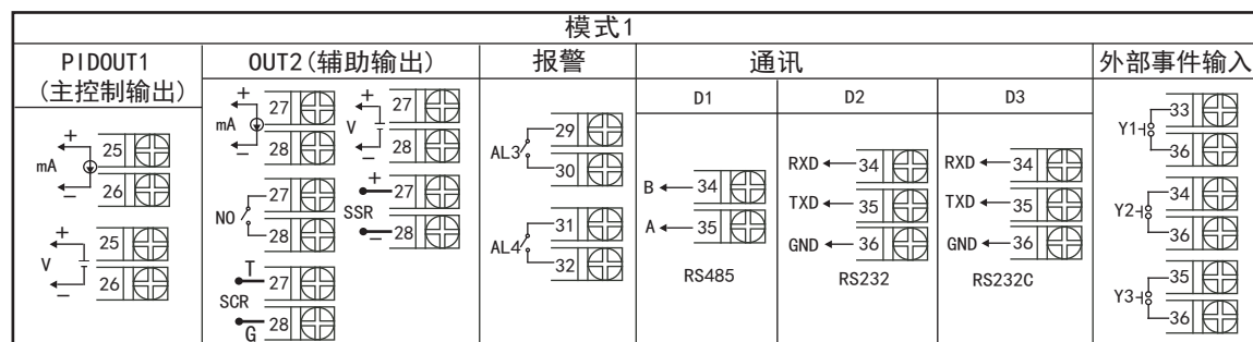
NHR-5330双路输入(阀位控制)PID温控器/调节仪接线图
