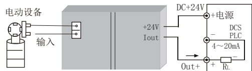
接线图二
