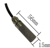
XHT03金属探头 特点：防尘、防水、响应灵敏
