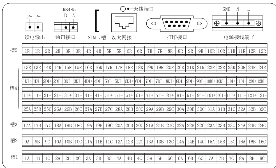
仪表尾部端子图
