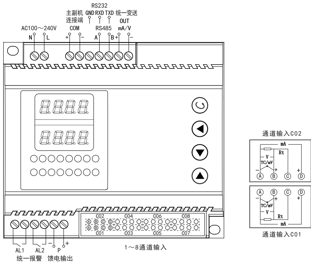
主机接线图
