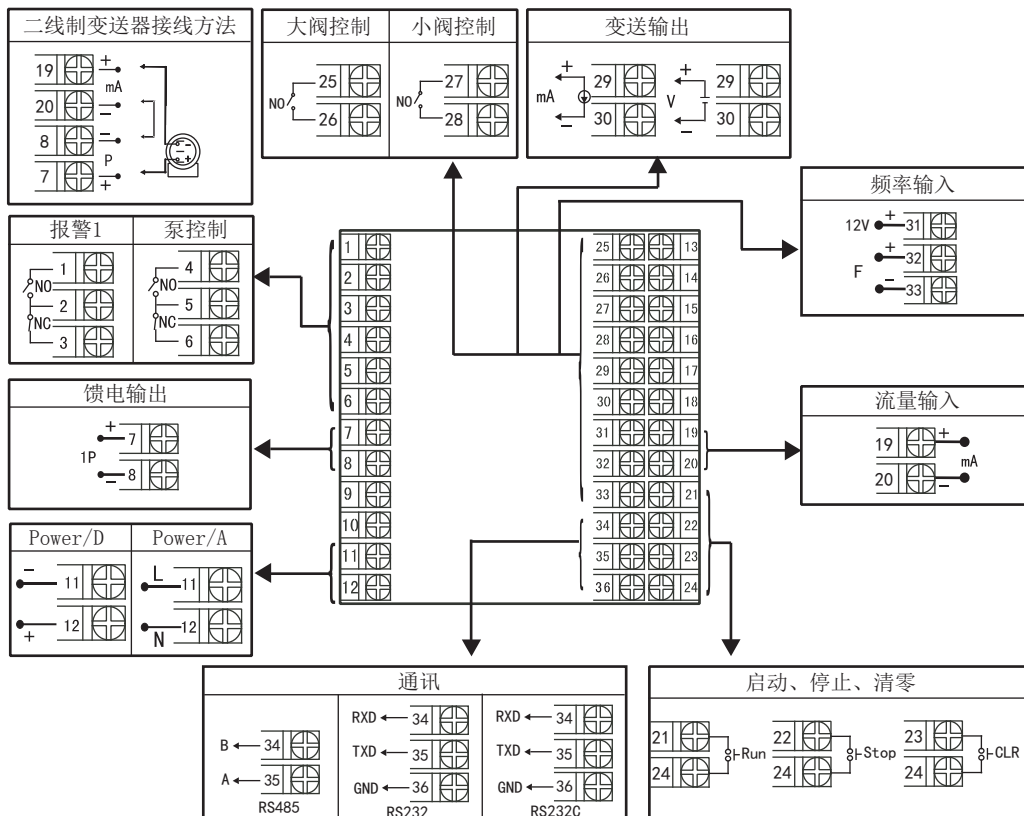
NHR-6671接线图
