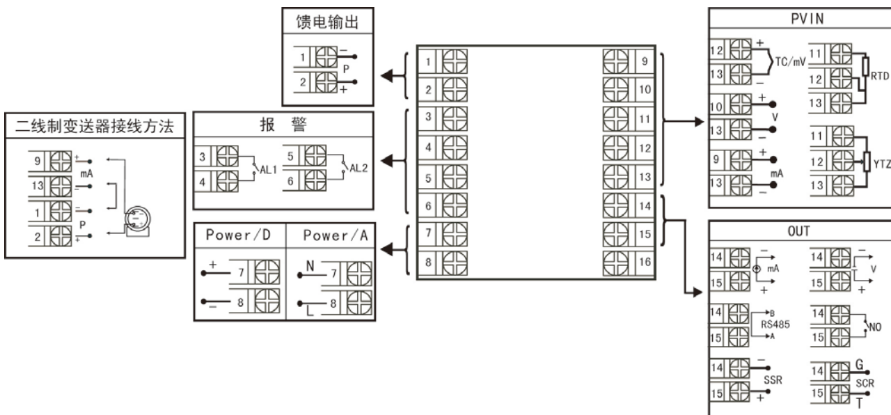
规格尺寸为 F 型接线图
