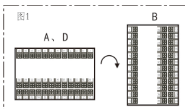
规格尺寸为 A、B、C、D 型接线图
