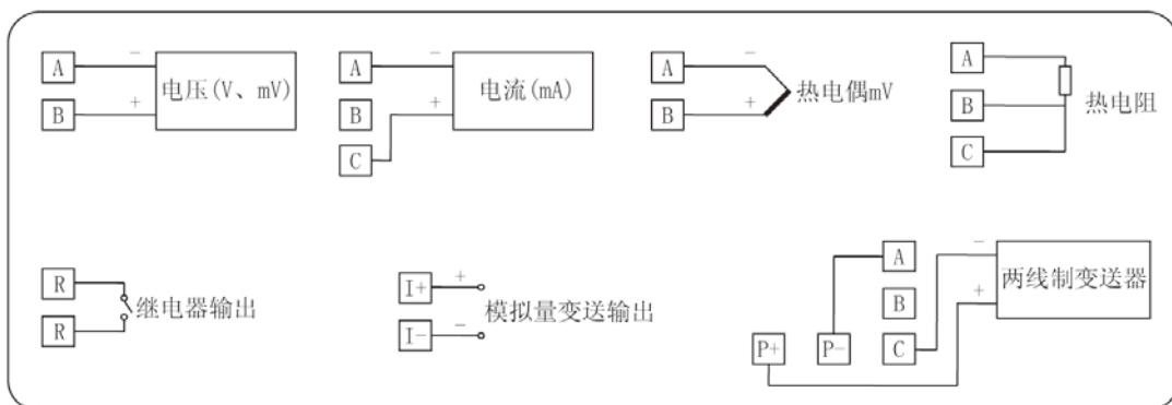
配线说明
