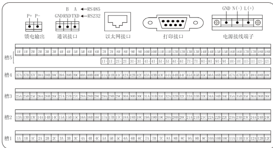
配线说明
