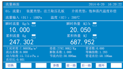
流量画面：将流量回路里的流量、温度、压力信息以组合的方式显示在同一画面上，同时显示各参数信息
