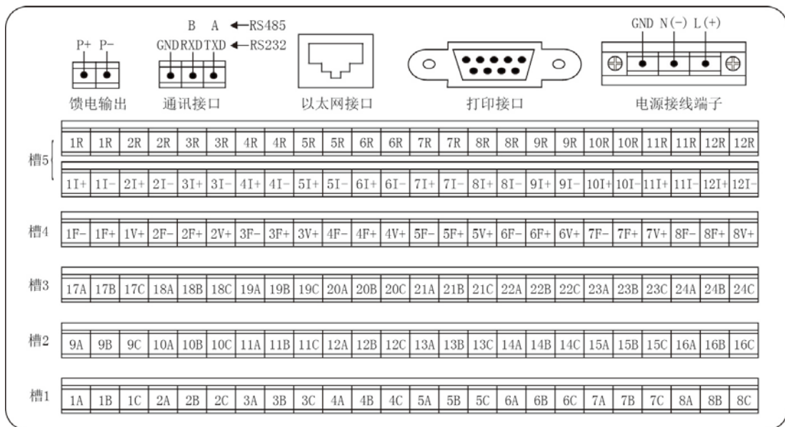
仪表尾部端子图
