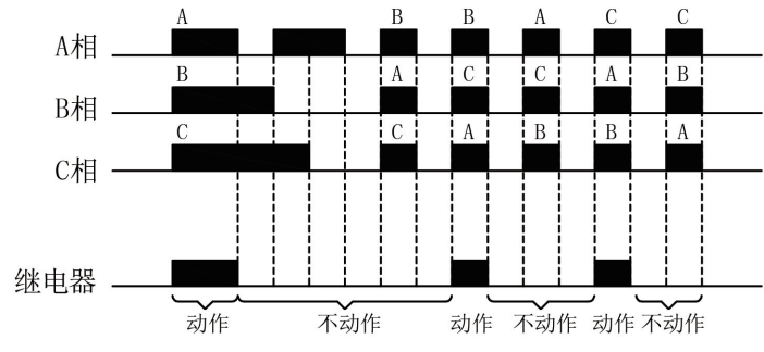
缺相监控时序图
