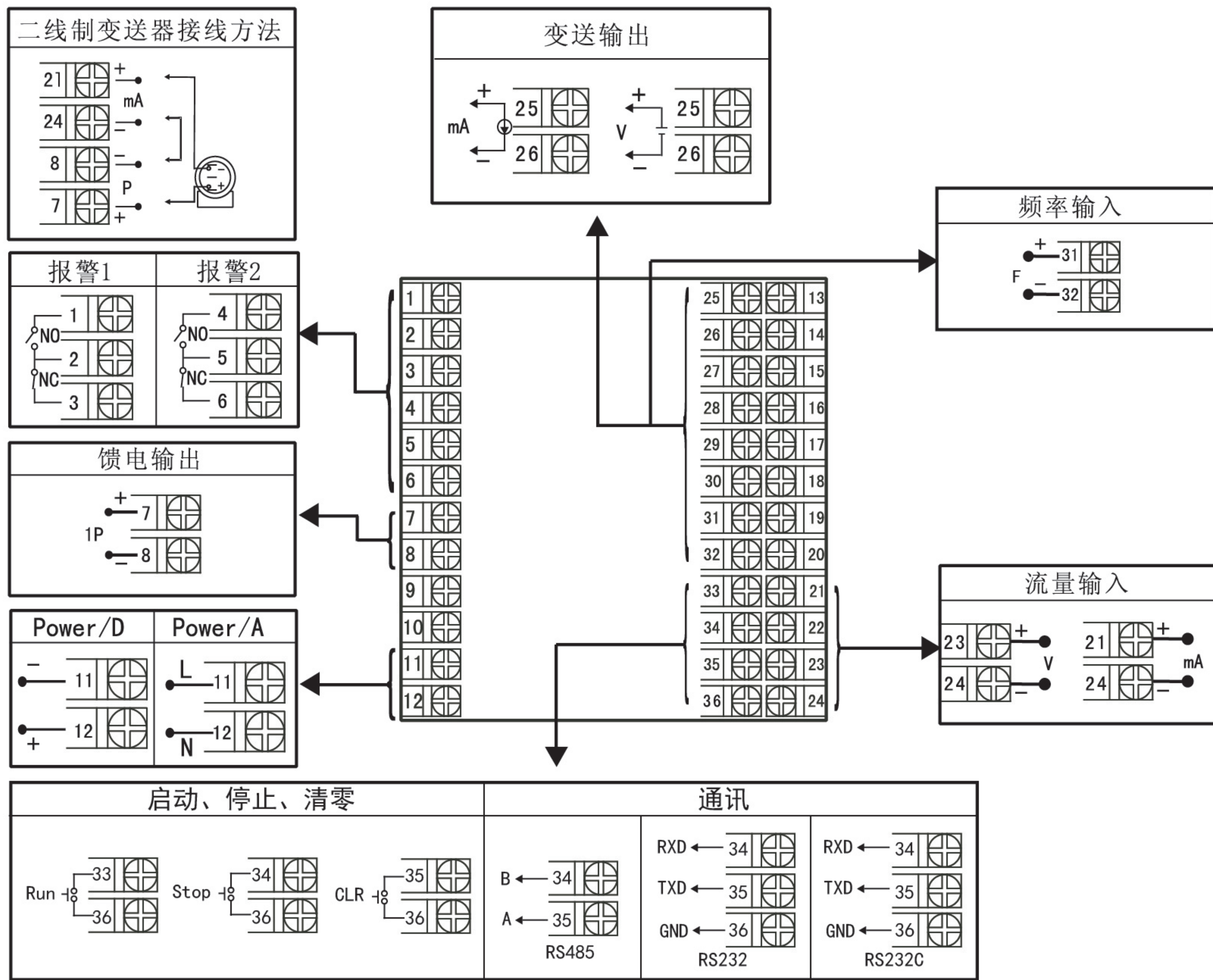
NHR-6602R接线图
