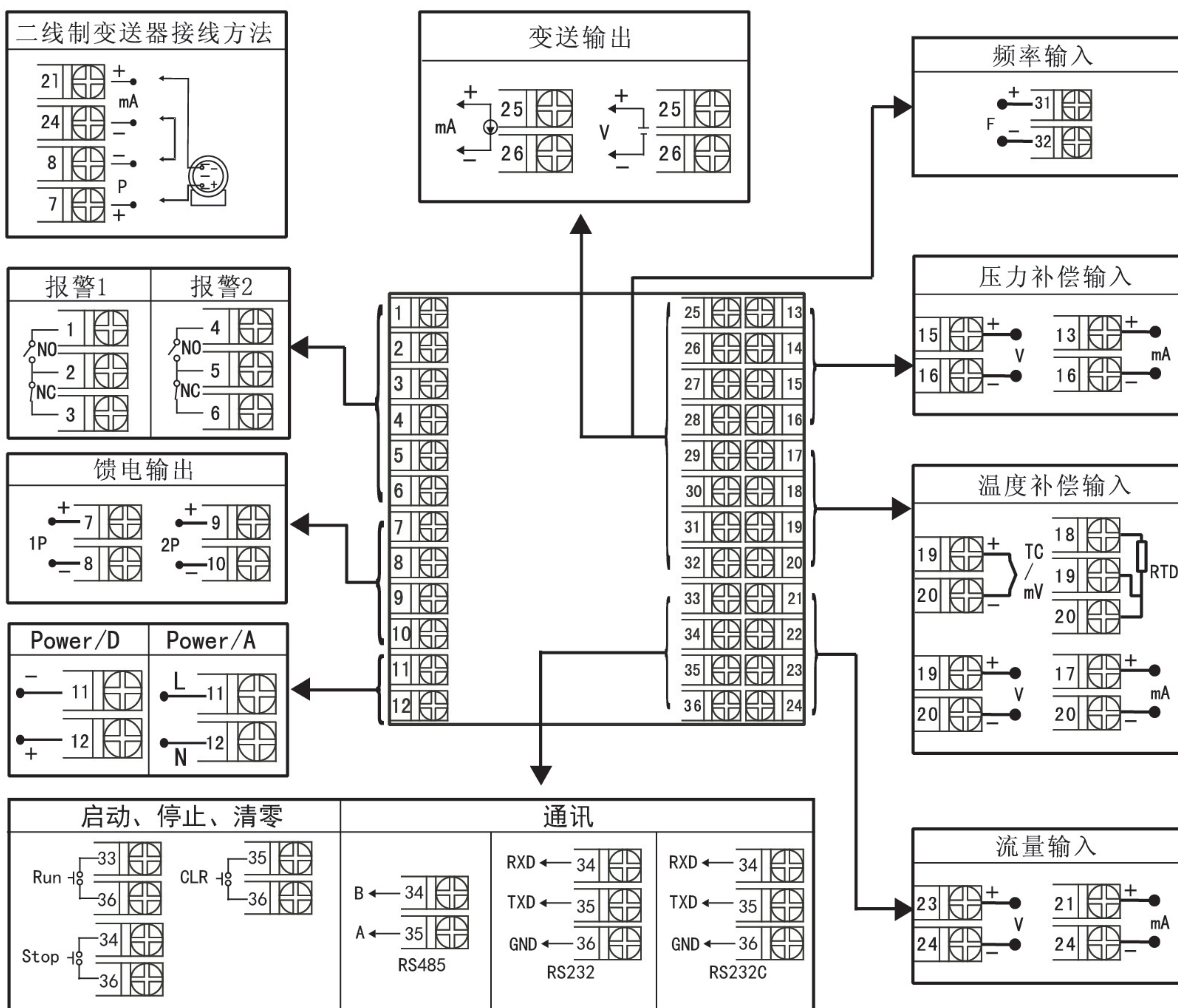
NHR-6602R接线图
