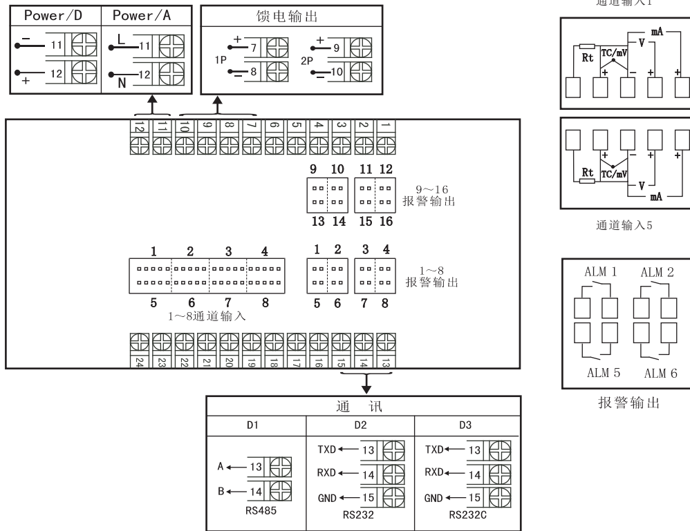
A、B型分别报警接线图
