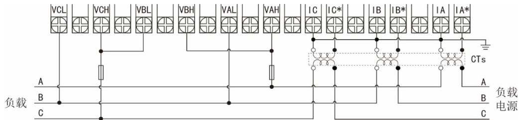
3-1-1、三相综合电量采用 CT 接入接线图 (适用于 3V3A)
