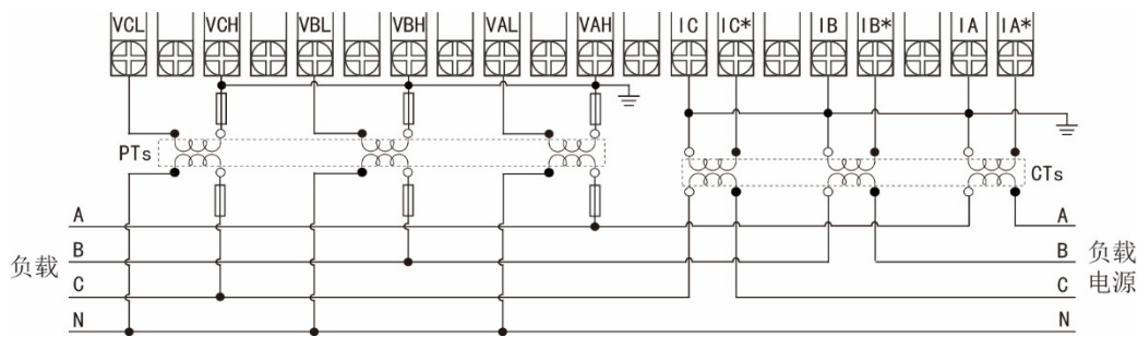
3-1-1、三相综合电量采用 CT 接入接线图 (适用于 3V3A)
