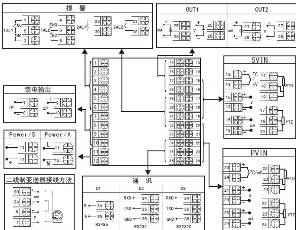
规格尺寸为 A、B、C、D、E、K、L、M 型接线图 注：横竖式仪表后盖接线端子方向不一样，见示意图 1
