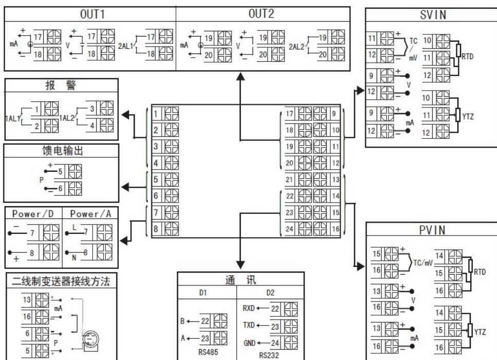
规格尺寸为 F 型接线图
