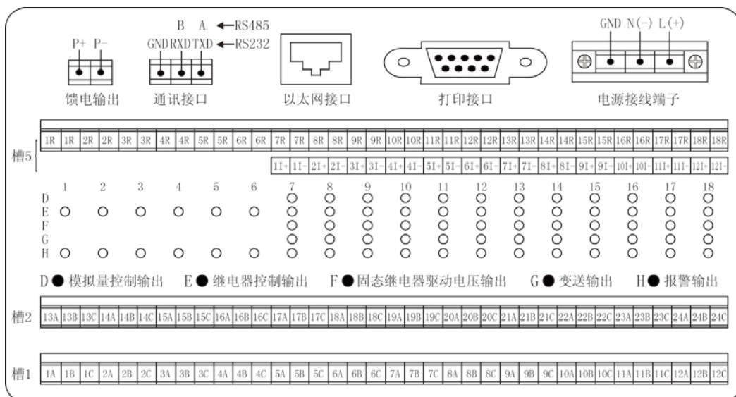
仪表尾部端子图
